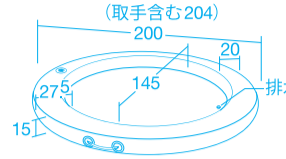
プール底面とフチ部分は、安全に配慮したすべり止め仕様。
